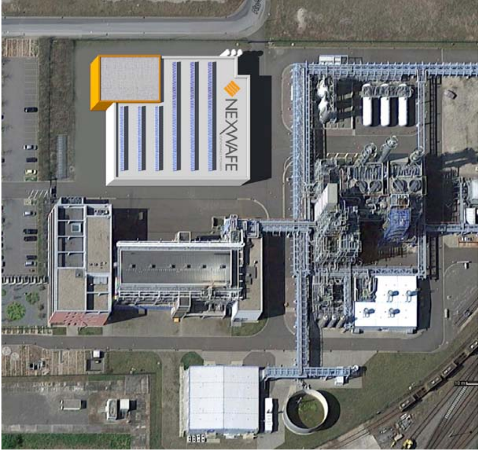
Werksgelände mit der geplanten Siliziumwafer-Fertigung
